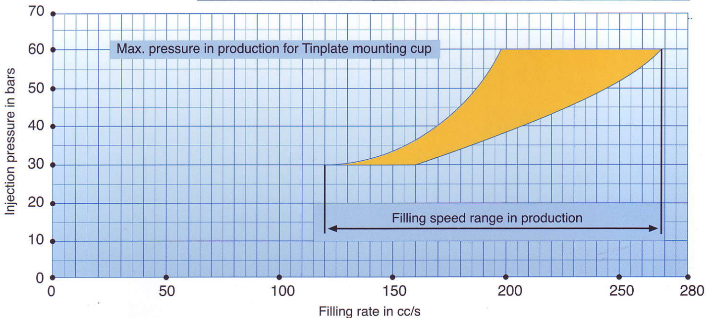
Filling Speed Diagram نمودار سرعت پرکن با استفاده از الوهای پادینه
